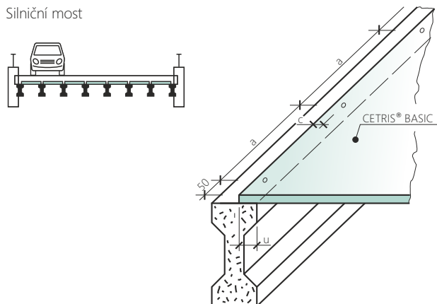
Silniční most
