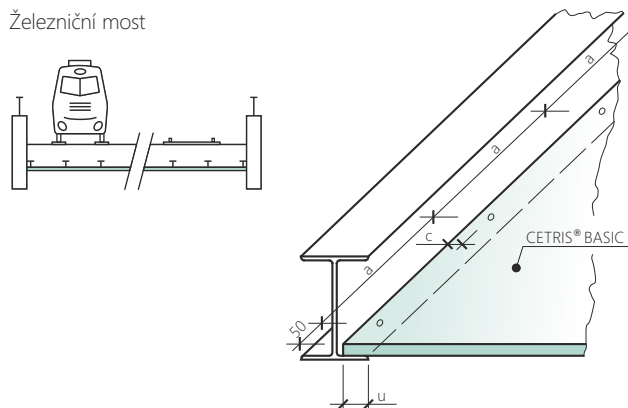
Železniční most
